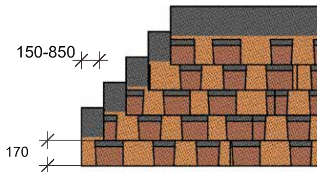
Рис. 4. Смещение гонтов ламинированной черепицы Döcke PIE DRAGON.
