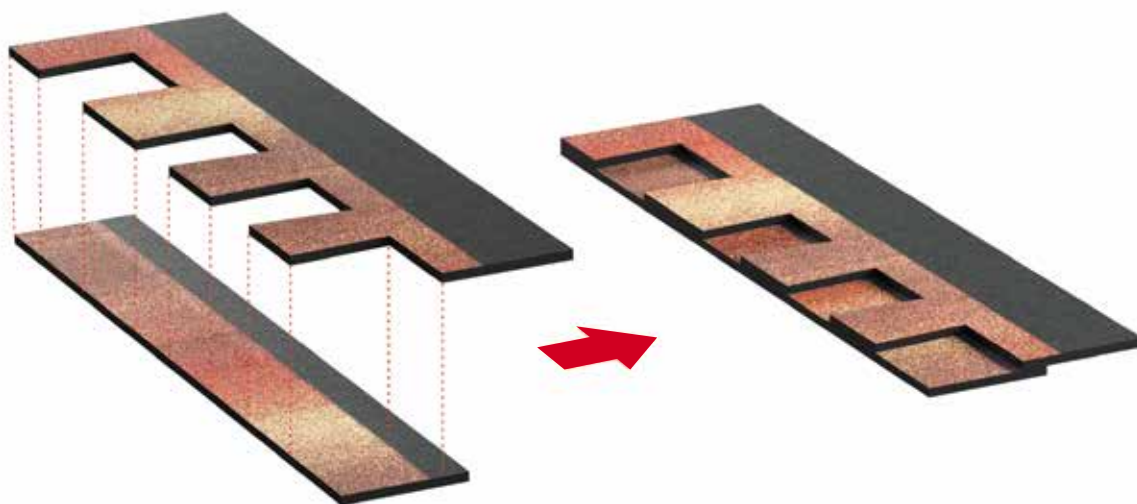
Рис. 1. Структура гонта ламинированной двухслойной черепицы.
